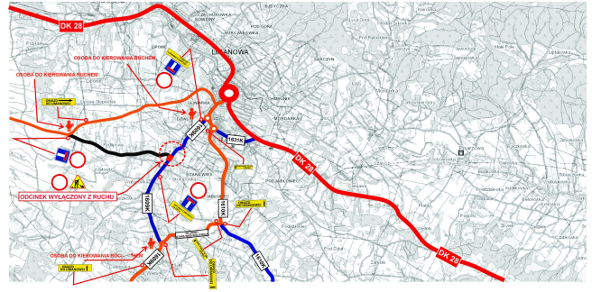
MAPA OBJAZDU NA CZAS ZAMKNIĘCIA ODCINKA DP 1609K ETAP II OD MOSTU W KM 1+670-2+250.
