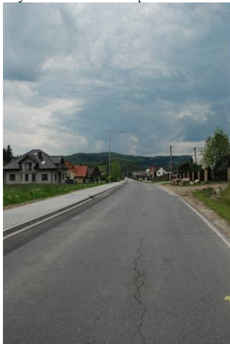
Rysunek 28 Zdjęcie inwestycji pn.: „Przebudowa odcinkowa drogi powiatowej nr 1615K Mszana Górna – Wilczyce w km 0+200 – 1+316 i w km 1+481 – 2+353 w miejscowości Mszana Górna/Łętowe poprzez wykonanie chodnika wraz z oświetleniem ulicznym – odcinek II.”
