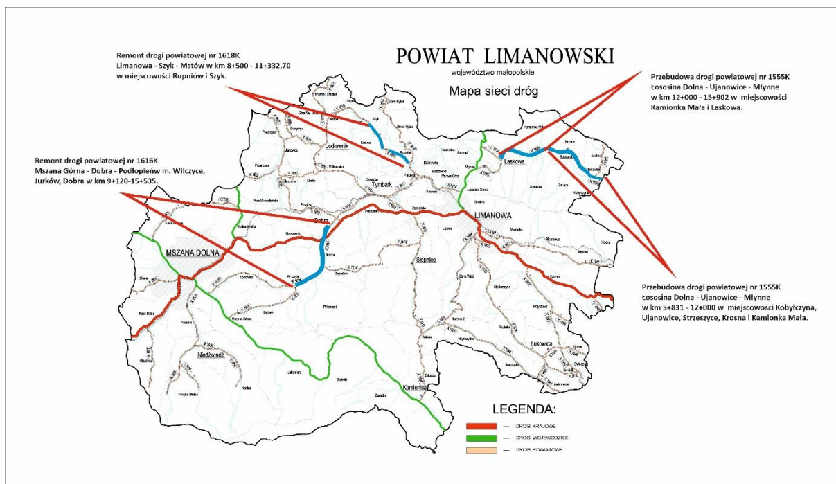
Rysunek 31 Dokumentacja projektowa.
